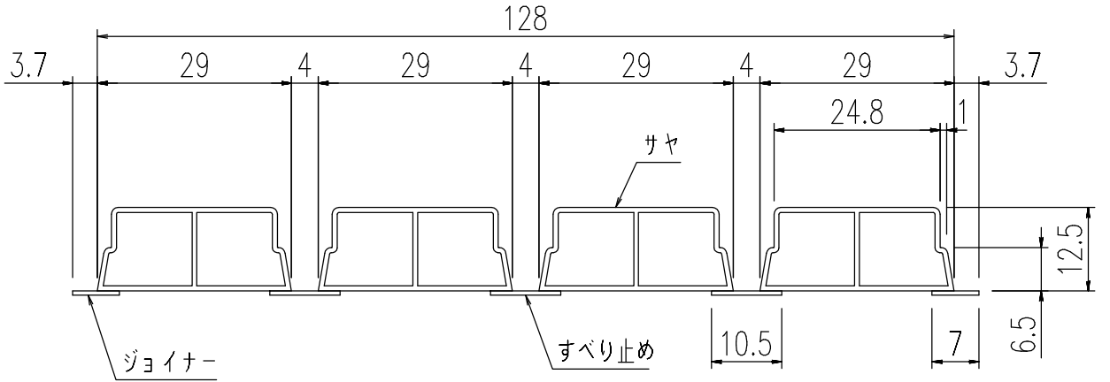
A-A' 断面図 (S=1/1)
