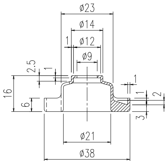
A-A'断面図
