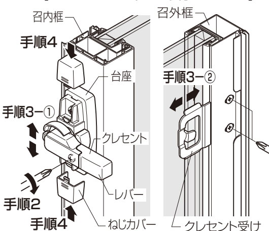
【ねじカバーを上下から取付けるタイプ】
