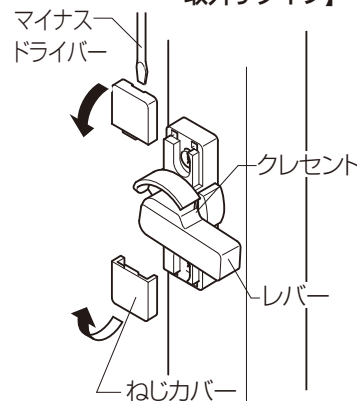
【ねじカバーを横に取外すタイプ】
