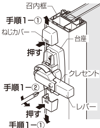
【ねじカバーを上下に取外すタイプ】
