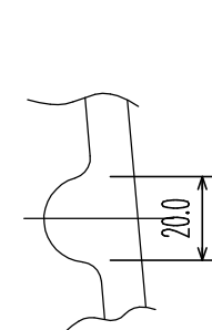
B部詳細(5/1)
