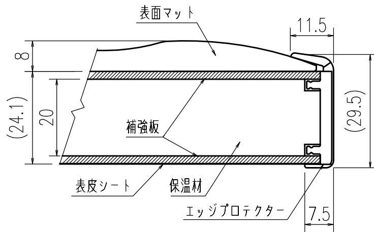
A-A 断面図 (S=1/1)
