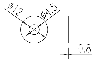
ワッシャー (S=1/1)
