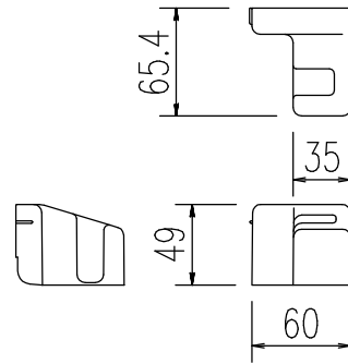
ダボカバー (S=1/1)
