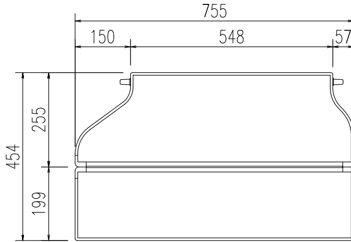
フタ本体 (S=1/10)
