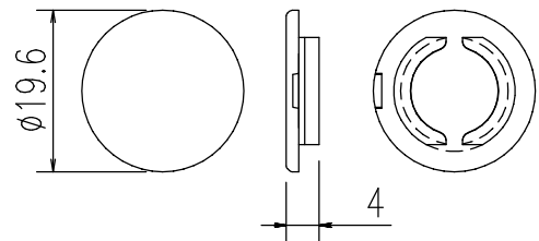
ダボカバー (S=1/1)
