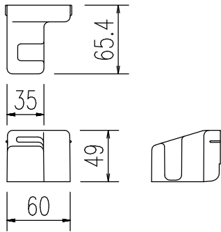
ダボ (S=1/1)
