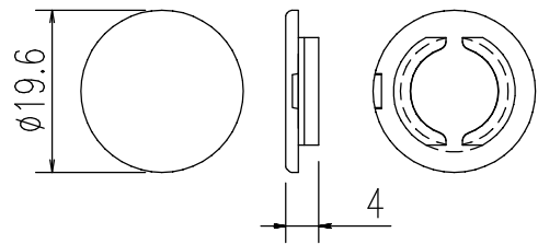
ダボカバー (S=1/1)
