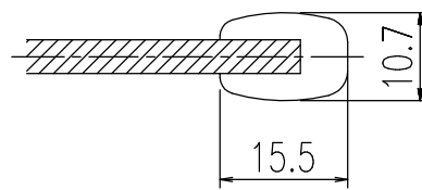
A-A 断面 (S=1/1)
