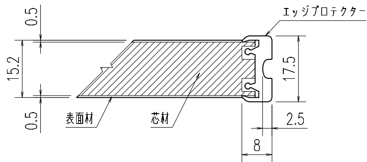
A-A断面図(S=1/1)
