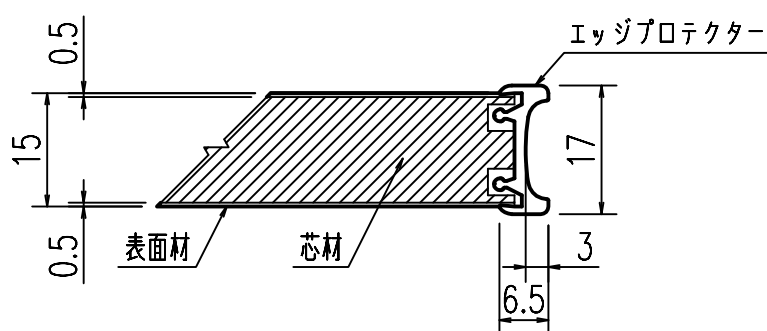
A-A断面図 (S=1/1)
