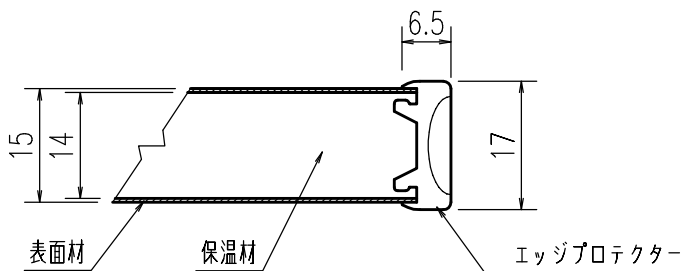
A-A 断面図 (S=1/1)
