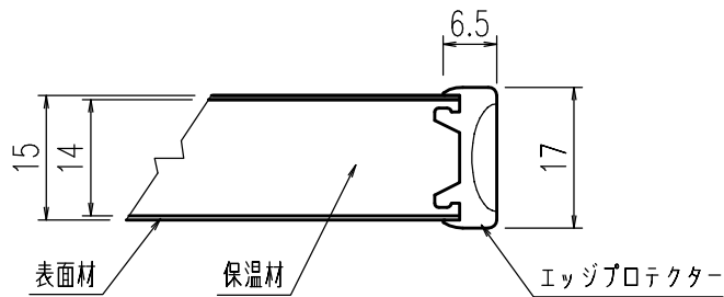
A-A 断面図 (S=1/1)
