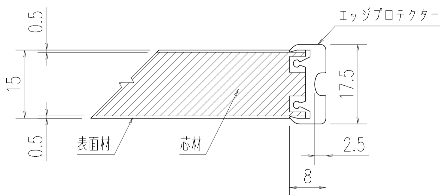
A-A断面図 (S=1/1)
