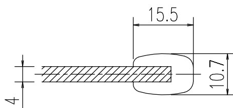
A-A 断面 (S=1/1)
