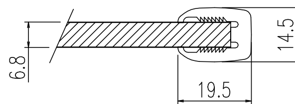
A-A'断面(1/1)
