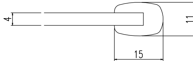
A-A'断面 S=2/1
