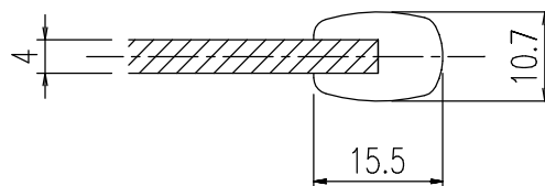
A-A 断面図 (S=1/1)
