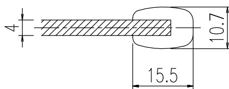
A-A断面 (S=1/1)
