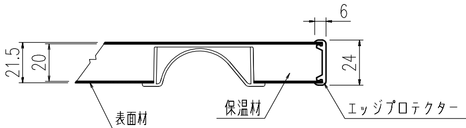
A-A断面図 (S=1/2)
