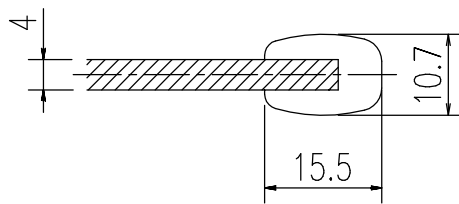
A-A断面 (S=1/1)
