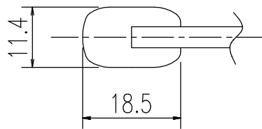
A-A断面図 (S=1/1)
