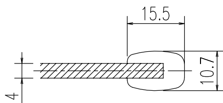
A-A断面 (S=1/1)
